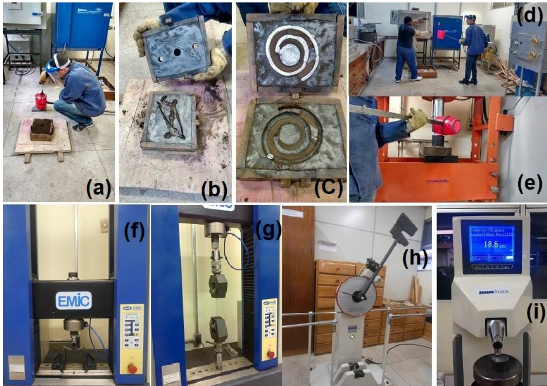
Figura 1 – Fotos das práticas relacionadas às disciplinas de Fundição e Ensaios dos Materiais. (a) Realizando retirada de escória pratica de fundição em areia verde, (b) Molde pronto para realizar vazamento, (c) Teste de fluidez em liga de alumínio, (d, e) squeeze casting, (f) Ensaio de flexão em 3 pontos, (g) ensaio de tração, (h) ensaio de impacto, (i) Ensaio de dureza Rockwell C. (Fonte: Autor)
